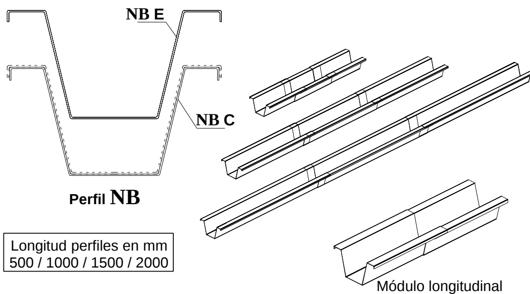
FIGURA 5. ESQUEMA DE PREFLECTADO
