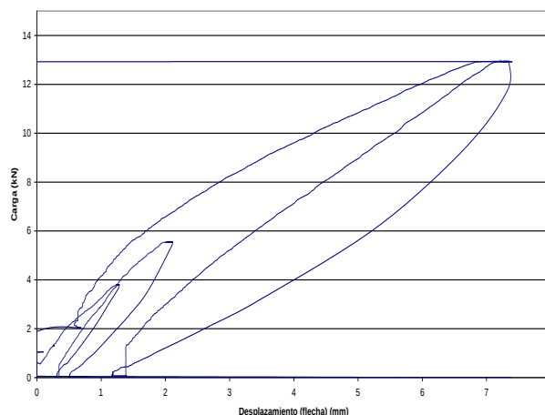
NOU BAU Ensayo forjado madera nº 1
