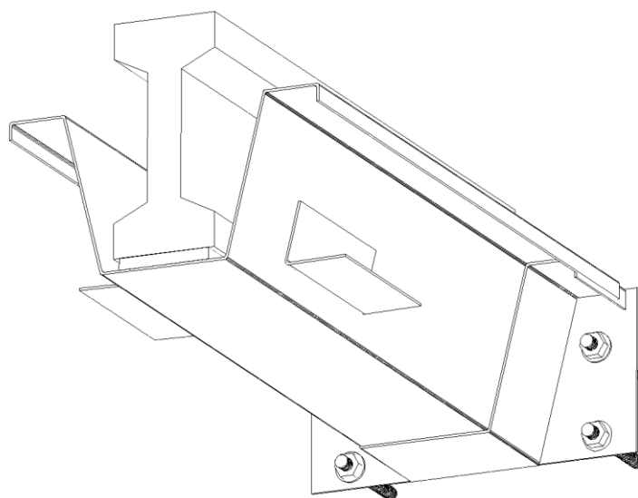
FIGURA 8. DISPOSICIÓN DE LOS ELEMENTOS COMPLEMENTARIOS
