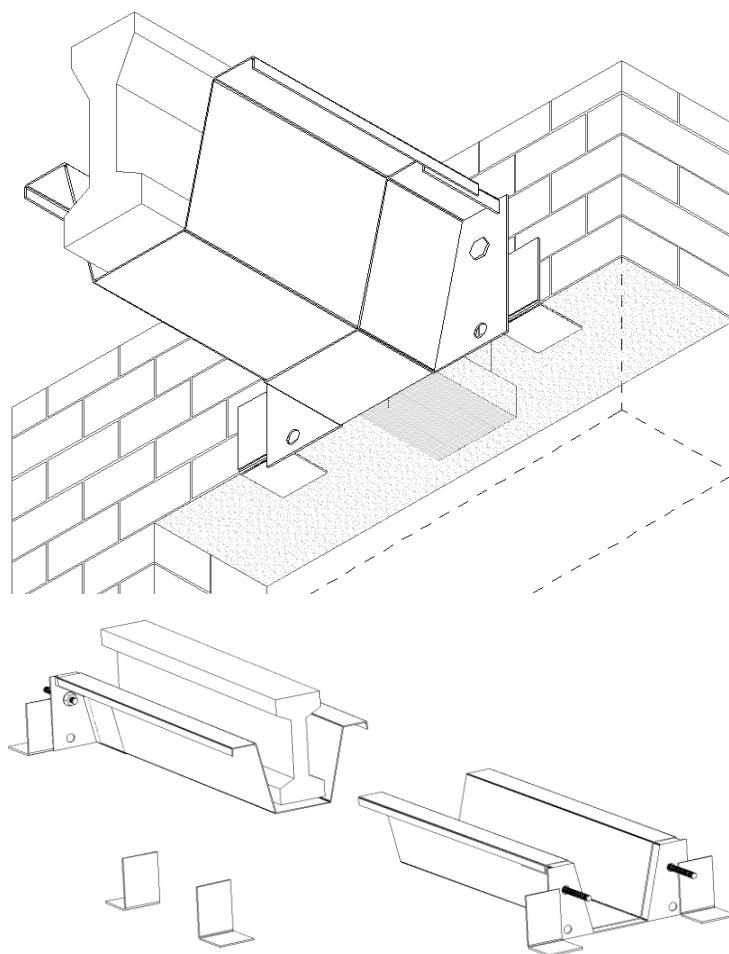
FIGURA 8. DISPOSICIÓN DE LOS ELEMENTOS COMPLEMENTARIOS
