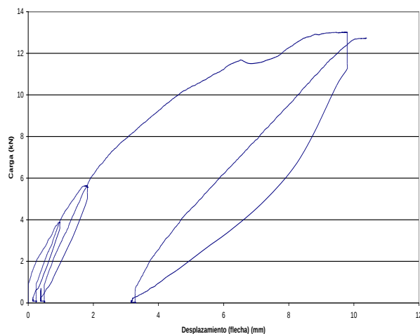
NOU BAU Ensayo forjado madera nº 2
